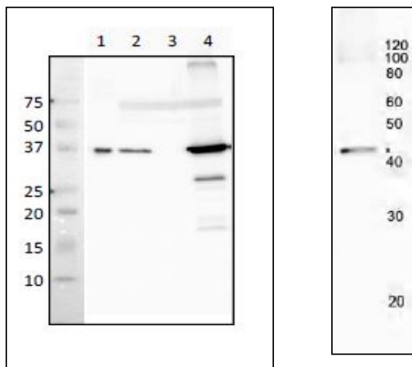
図 1. E. coli の粗抽出液中の RecA タンパク質のウェスタンブロット法による同定。レーン 1; 精製 RecA 8 ng. レーン 2, 野生型株粗抽出液. レーン 3、recA 欠失株粗抽出液. レーン 4; lexA 欠失株 (SOS 遺伝子を過剰発現)粗抽出液. 抗体は、1/3,000 の希釈で使った。細胞抽出物, 2 \mu g
