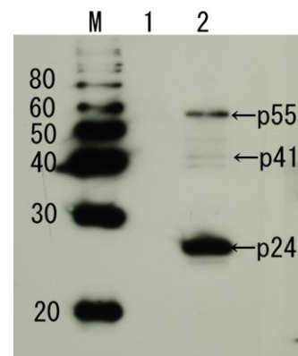
図 1 抗 HIV-1 p24 抗体を用いたウエスタンブロット法による p24 抗原の検出 レーン 1 : MT4 細胞抽出液 レーン 2 : HIV-1 (LAI 株)感染 MT4 細胞抽出液 抗血清は 2,500 倍希釈して使用
